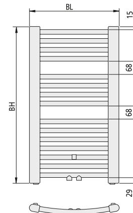
Vorderansicht
