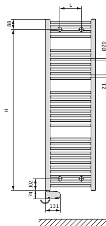
Rückansicht
